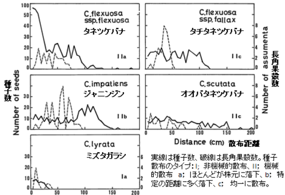
図 3.2. 種子散布
